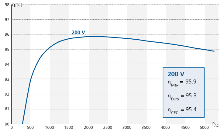
Wirkungsgradkennlinie Powador 6002
